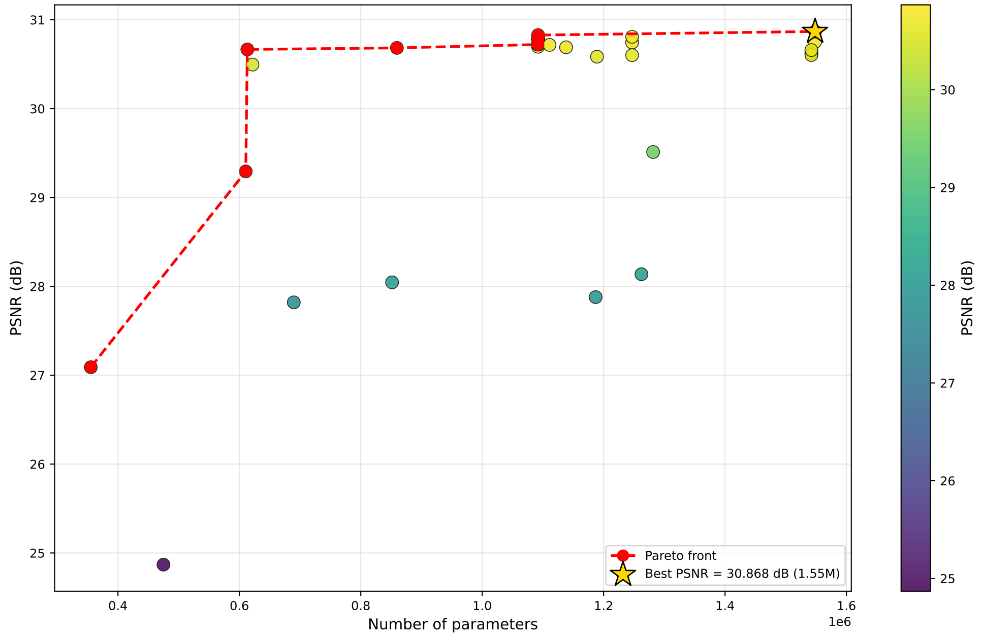
PSNR vs #Parameters — HAT
